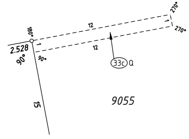
ENLARGEMENT 'F2' SCALE 1:200
