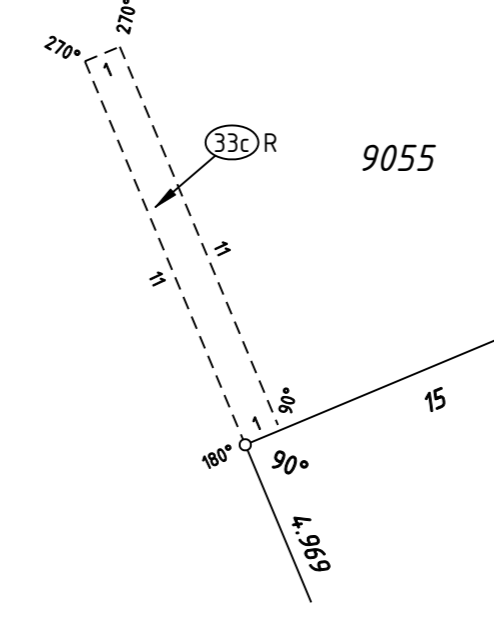
ENLARGEMENT 'G2' SCALE 1:200
