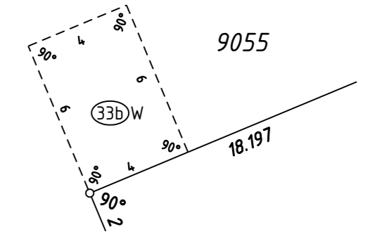
ENLARGEMENT 'H1' SCALE 1:200
